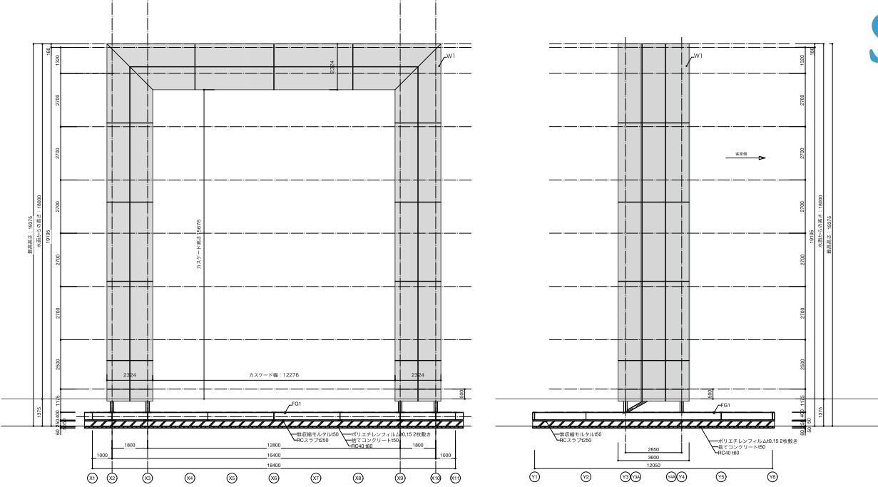
オブジェ最終図面。スクリーンとなる投影面には、水を下に落とすためのウォーターカスケードを使用している。
